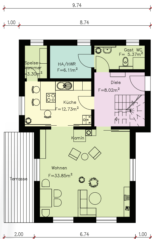
Grundriss Erdgeschoss
