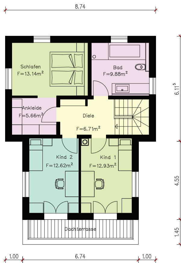
Grundriss Dachgeschoss
